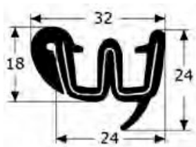
GC400 Ventanilla corredera (3,30 m)
